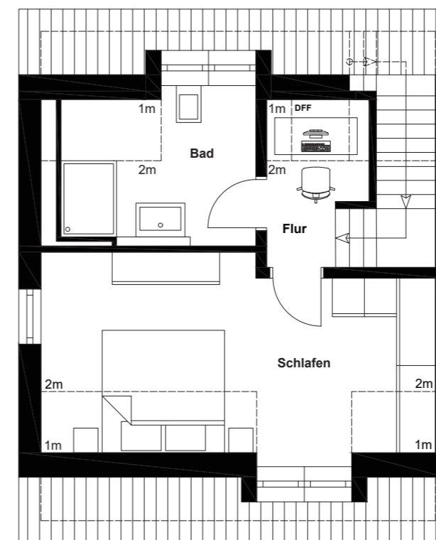
DACHGESCHOSS
