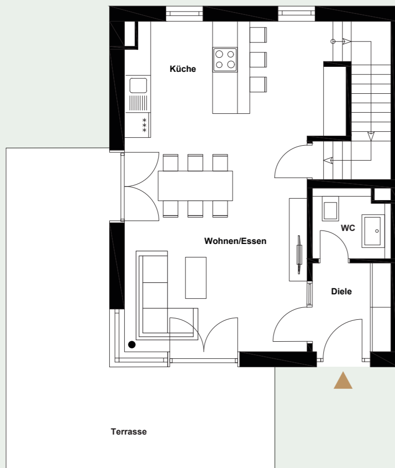
ERDGESCHOSS
