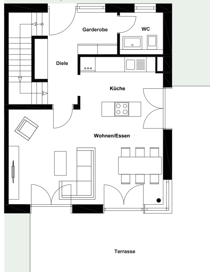
ERDGESCHOSS
